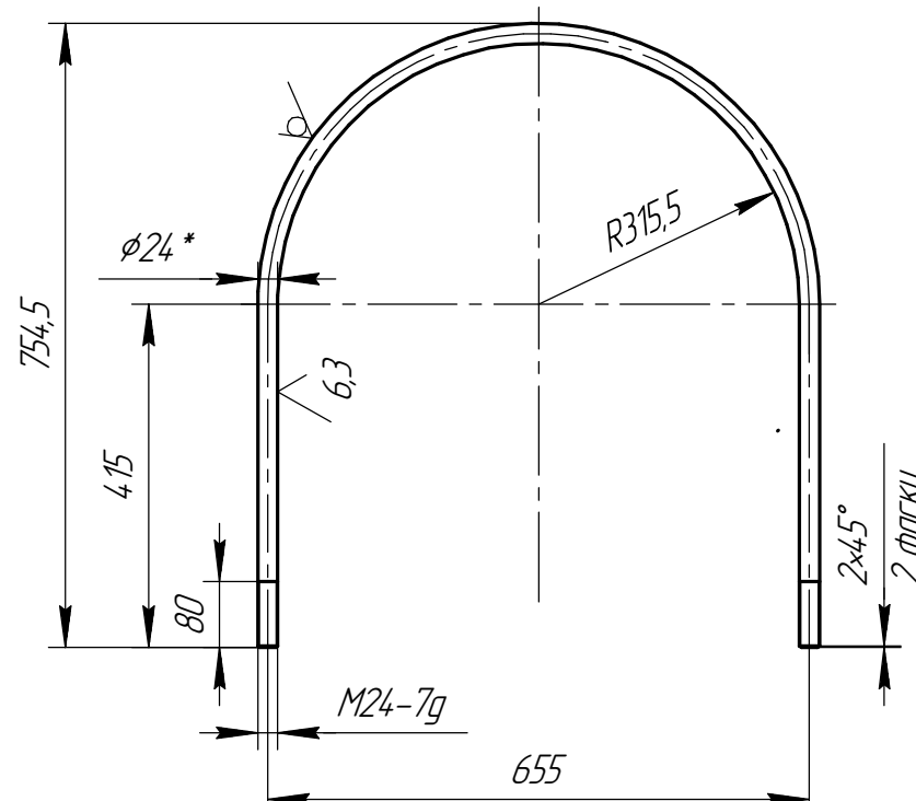
Дет. поз. 5 (1:10)
