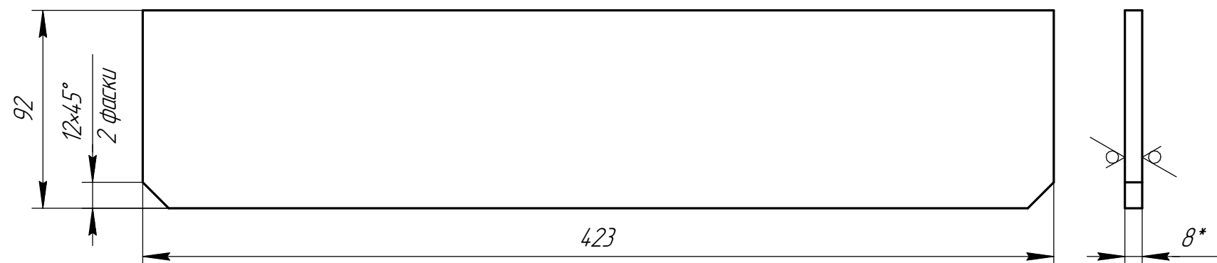
Дет. поз. 2 (1:2,5)
