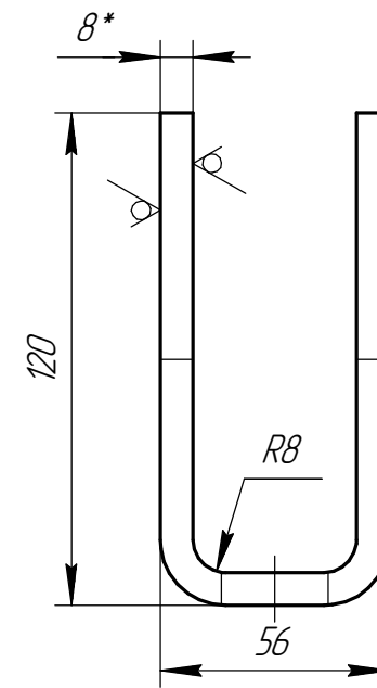
Дет. поз. 3 (1:2)
